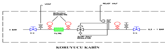
Şekil - 6 İkincil basınç düşürme istasyonu
