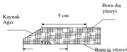
Şekil-7 Kaynak ağızı
