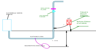
Şekil-17 Galvanik anotlu katodik koruma sistemi
