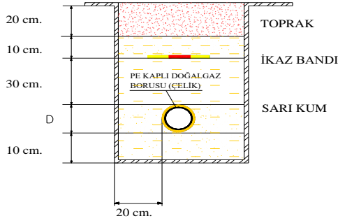
Şekil-1 Çelik boru hatlarına ait tranşe detayı
